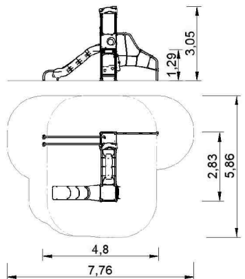
Multijuego Veleta doble Double Veleta playset Structure multi-jeux Veleta double
