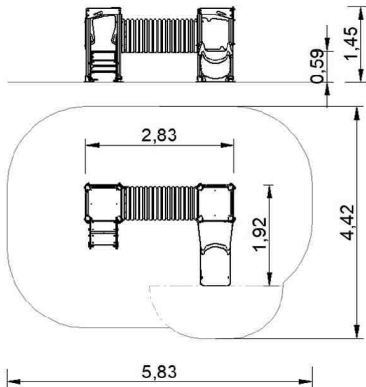
Veleta gateador Crawling Veleta Veleta Tunnel à Ramper
