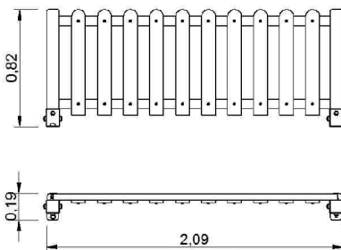
Valla Veleta Veleta Fence Clôture Aire de Jeux Veleta
