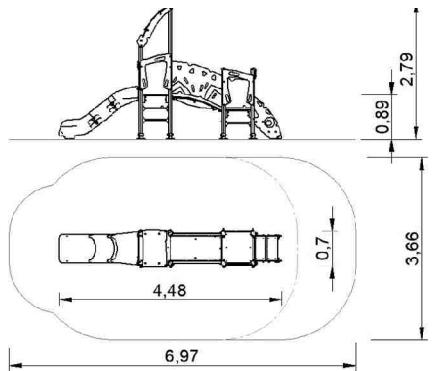
Veleta en línea Lined Veleta Veleta en Ligne Droite
