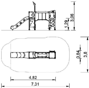
Multijuego Gran Veleta Great Veleta playset Structure multi-jeux Grand Veleta
